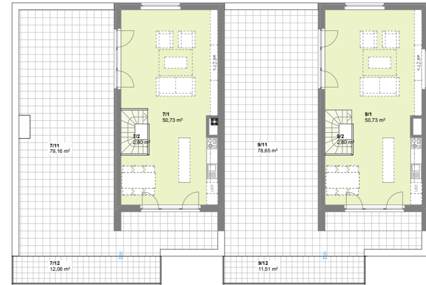
Púdorys 4.NP
