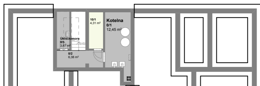
Púdorys 1.PP
