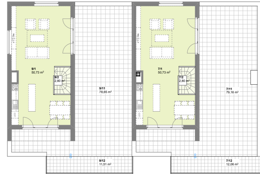
Půdorys 4.NP
