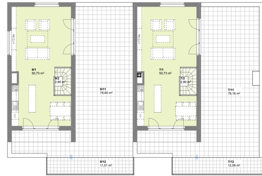
Púdorys 4.NP
