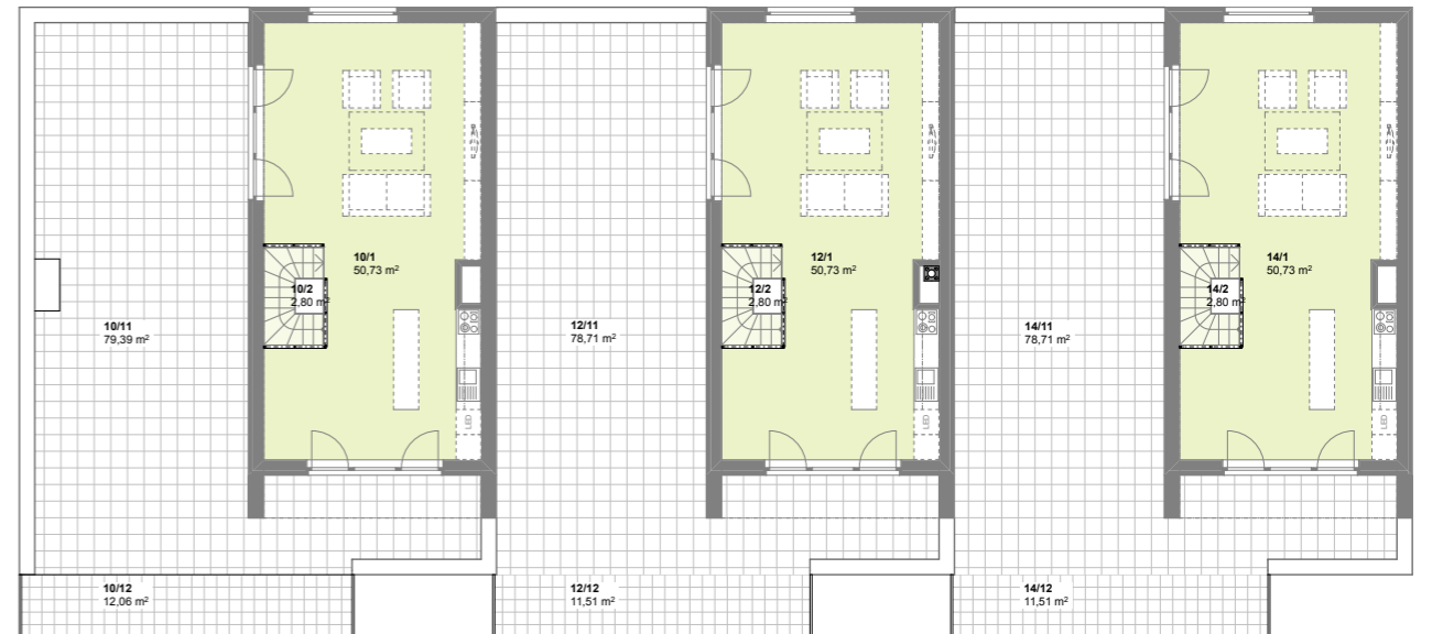
Púdorys 4.NP
